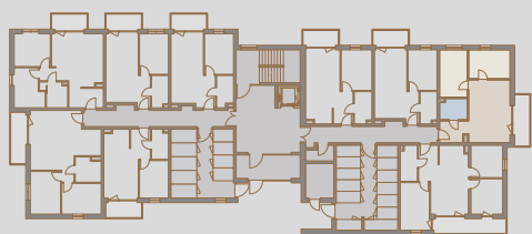
RZUT KONDYGNACJI
